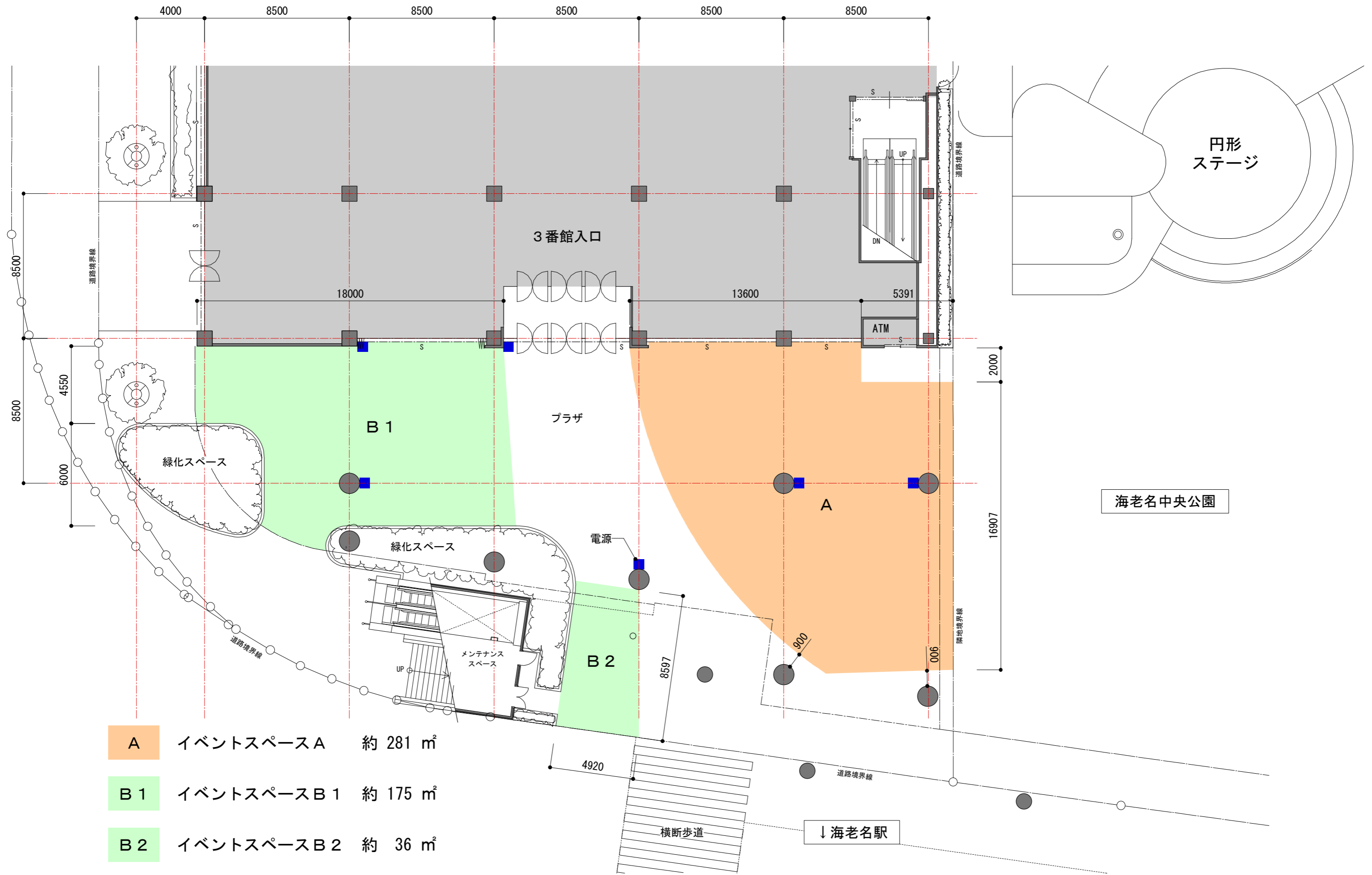
ビナウォーク 3番館1F ビナプラザ平面図 S=1/200
